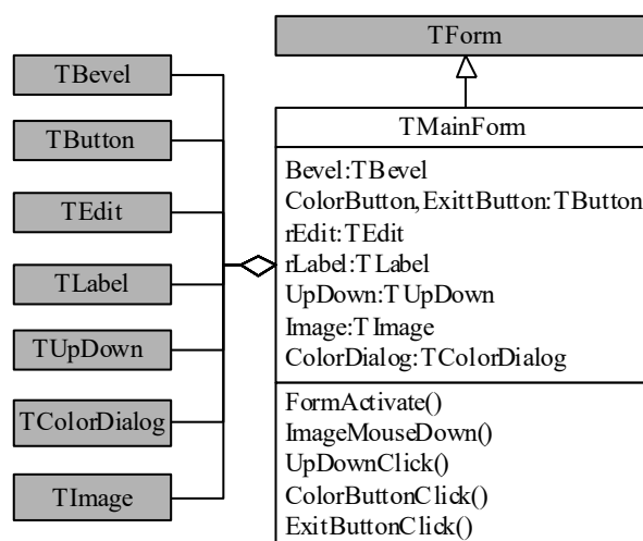
Рисунок 11 - Диаграммы классов предметной области ( a ) и интерфейсной части ( b )
