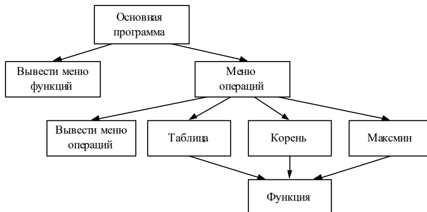
Рисунок 9 - Структурная схема программного продукта (процедурная декомпозиция)
