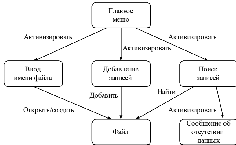
Рисунок 8 - Структурная схема программного продукта (объектная декомпозиция)
