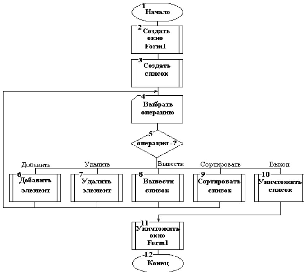
Рисунок 10 - Алгоритм основной программы (процедурное программирование)
