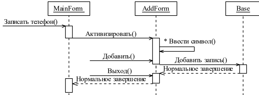
Рисунок 12 - Диаграмма последовательности действий
