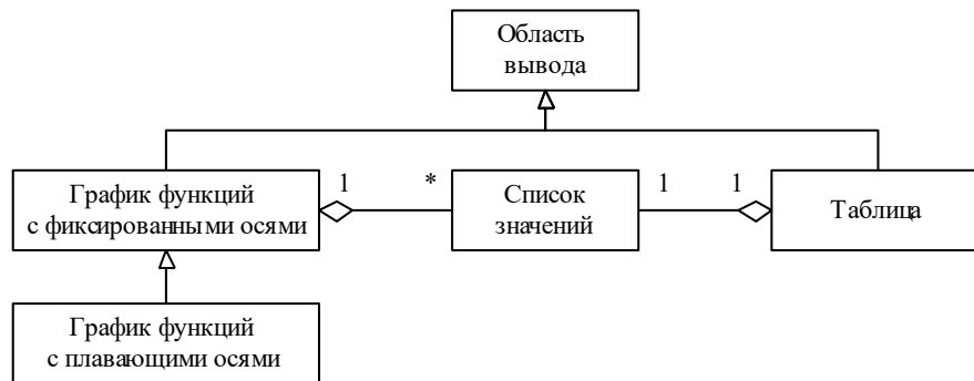
Рисунок 2 - Концептуальная диаграмма классов
