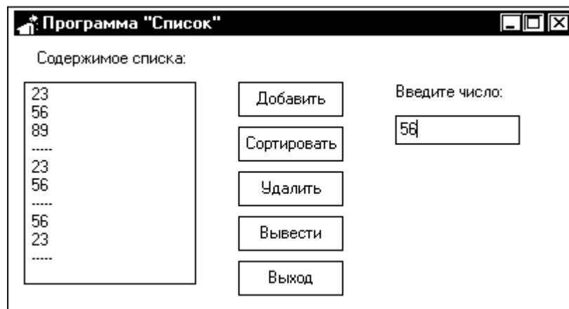
Рисунок 4 - Экранная форма
